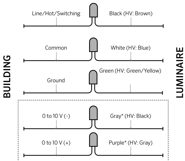
Wiring Chart
